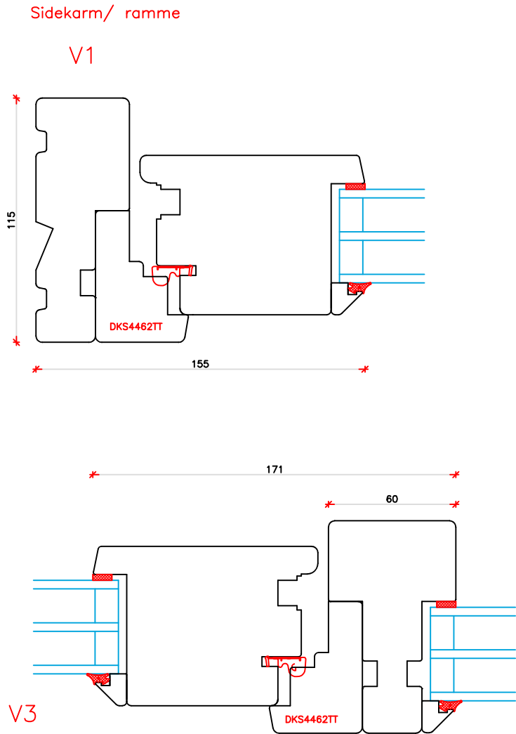
Lodpost/ ramme
