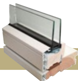
Udvendig profil, 2 lags glas
