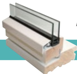
Udvendig profil, 2 lags glas
